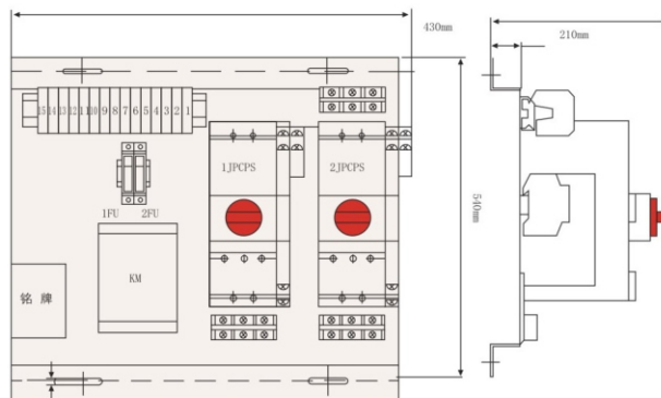
JPCPSD-100 外型尺寸
