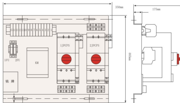
JPCPSD-45 外型尺寸
