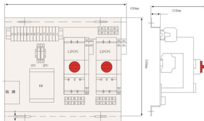
JPCPSN-100 外型尺寸
