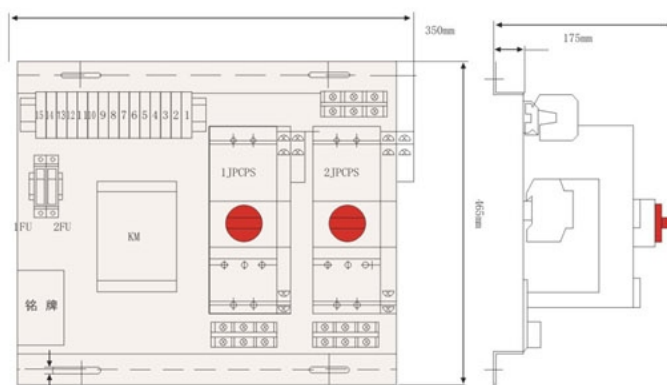
JPCPSN-45 外型尺寸
