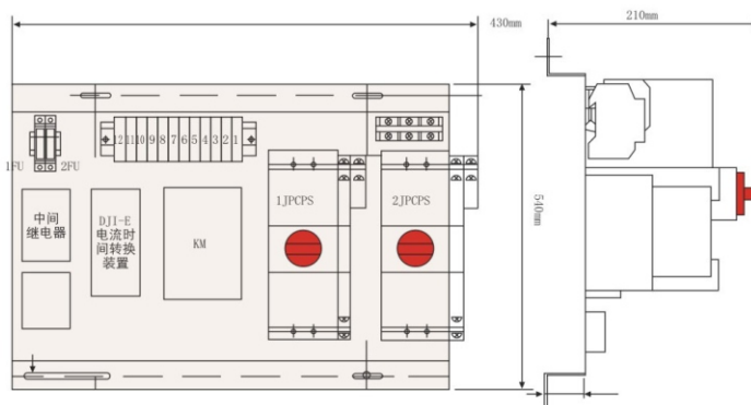
JPCPSZ-100 外型尺寸
