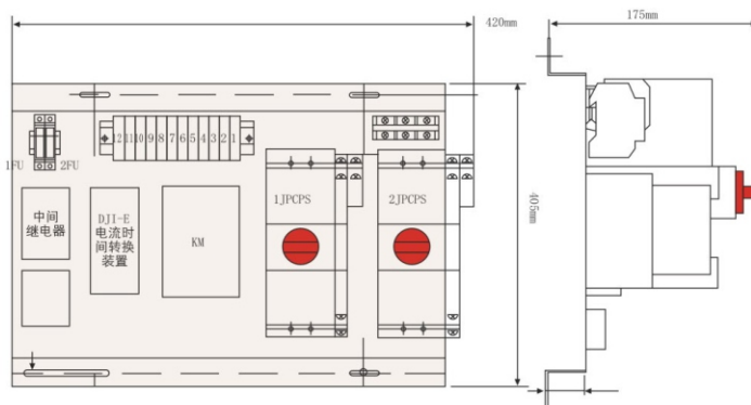
JPCPSZ-45 外型尺寸
